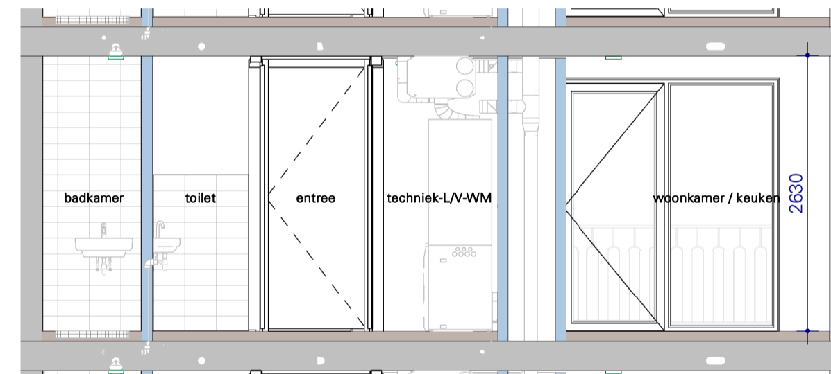
VK Doorsnede B - Blok E -bnr099
